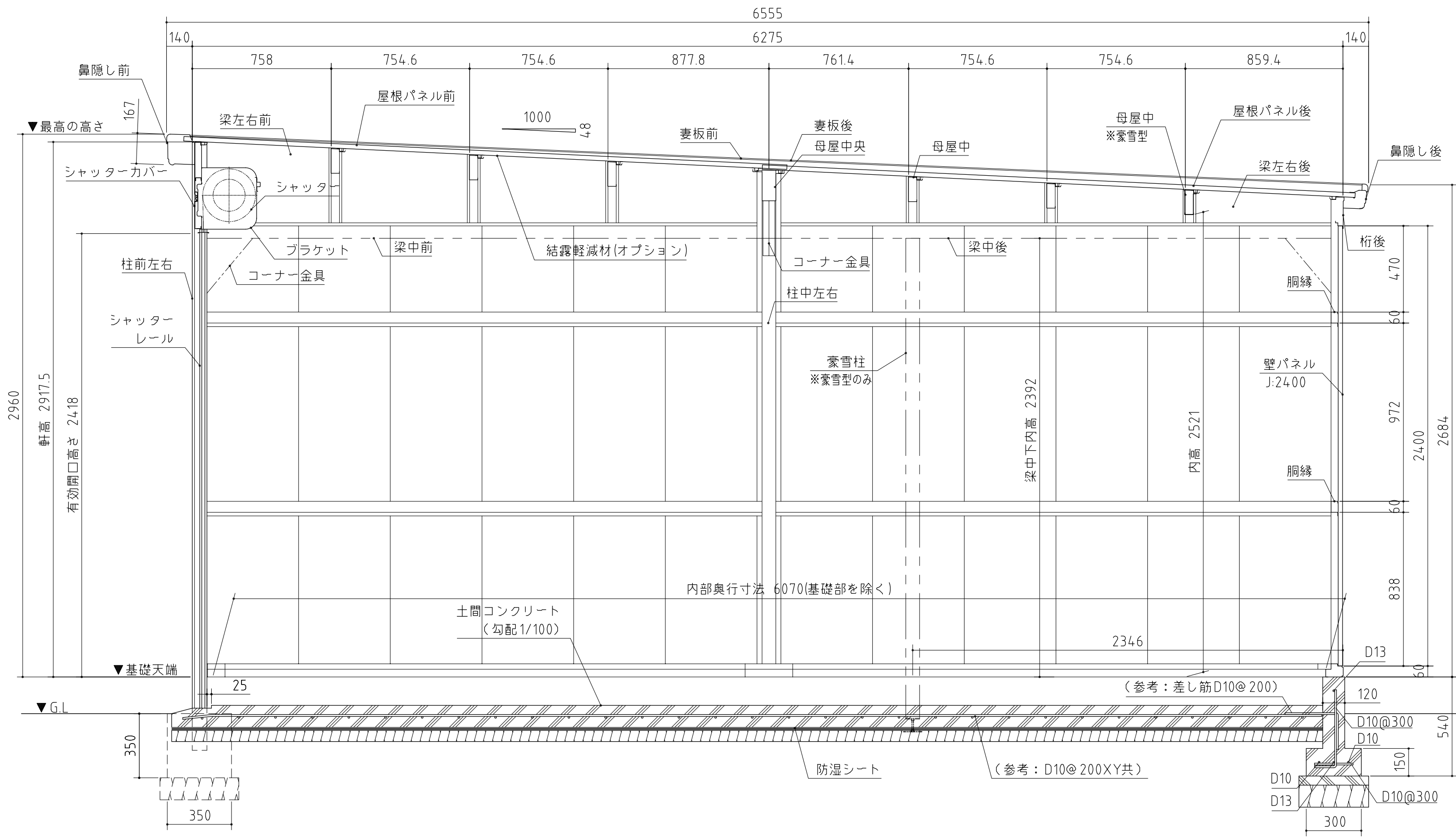
断面図(側面) <縮尺> S=1/20 ~一般型・豪雪型~ 機種名 GRN-2662J・JL、3162J・JL 3662J・JL
